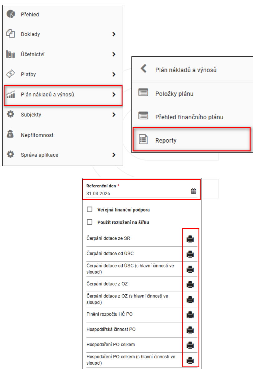
Obrázek 23: Zobrazení Reportů
